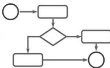
Рисунок 1.Образец блок-схемы
